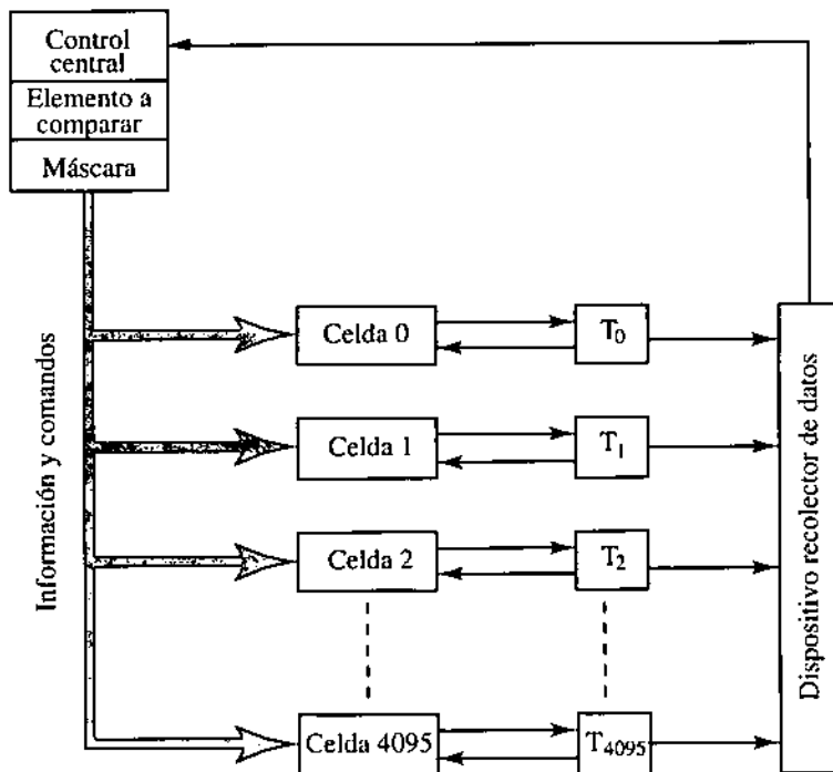
Figura 7.32 • Revisión de una memoria asociativa (adaptado de Foster).
