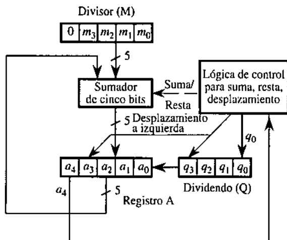
Figura 3.14 • Circuito divisor serie.
